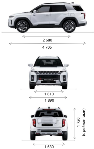
Размеры, мм
